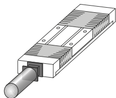
Spindelantrieb mit stirnseitigen Motoranbau
