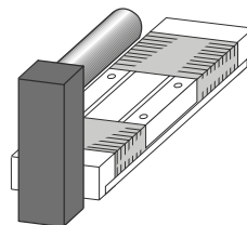
Spindelantrieb mit Motoranbau oben
